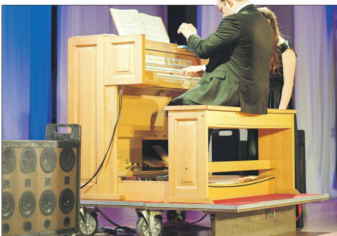
Как видите, игровой пульт цифрового органа ничем не отличается от пультов духовых органов. Но вместо труб к нему подключена компьютерная система, каждый звук с которой записан с тысяч труб настоящего органа
